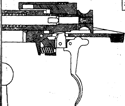
後膛機全部分剖面
