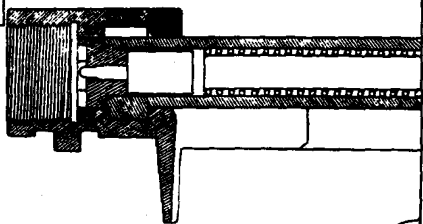
復膛機全部分割面
