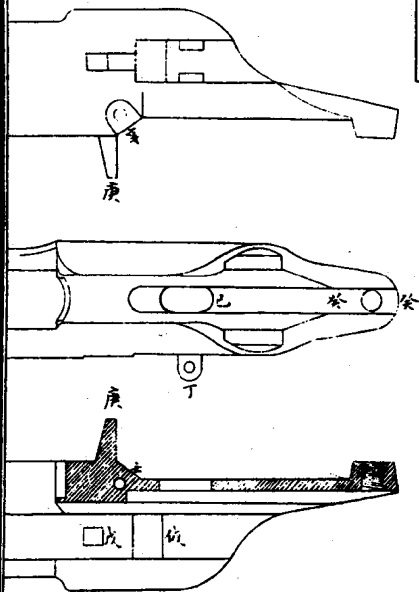
槍圖一 槍槍
