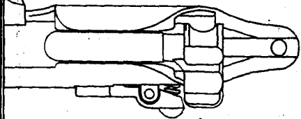
後膛機全部分剖面
